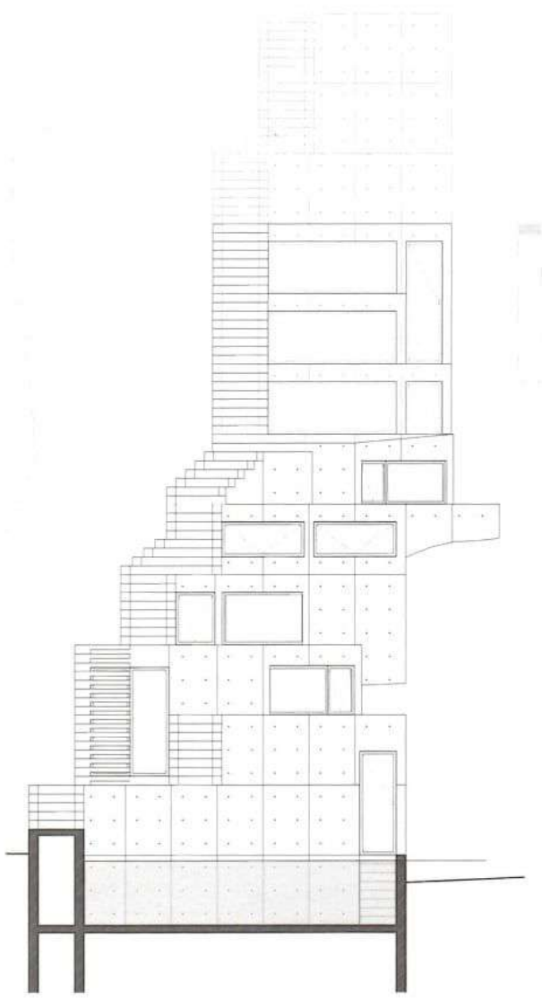
Sección JJ'
