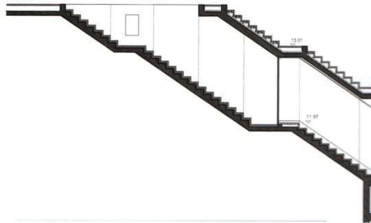
Sección NN'
