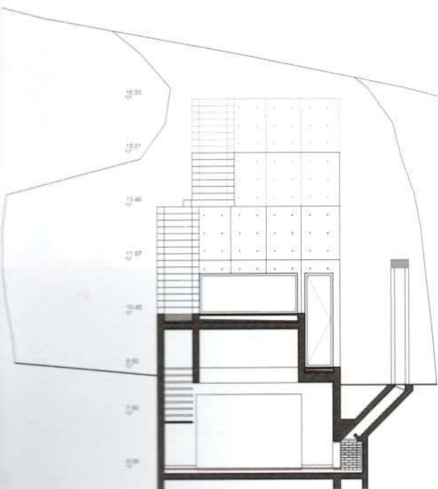
Sección BB'
